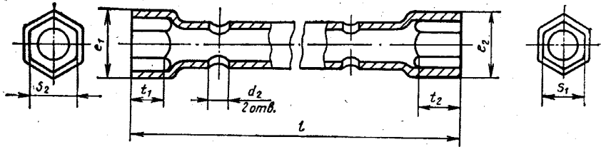
Исполнение 2
